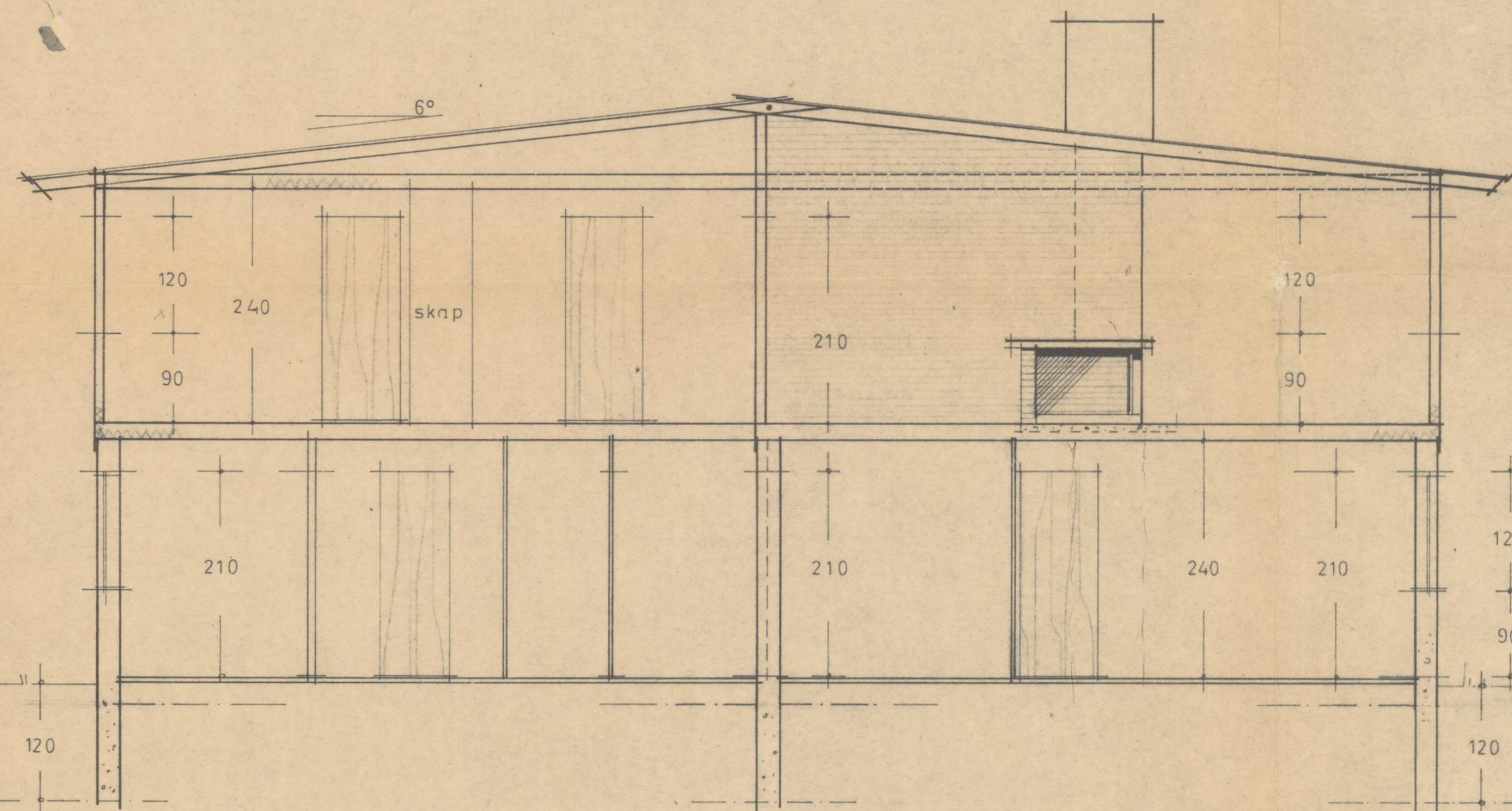
SNITT
