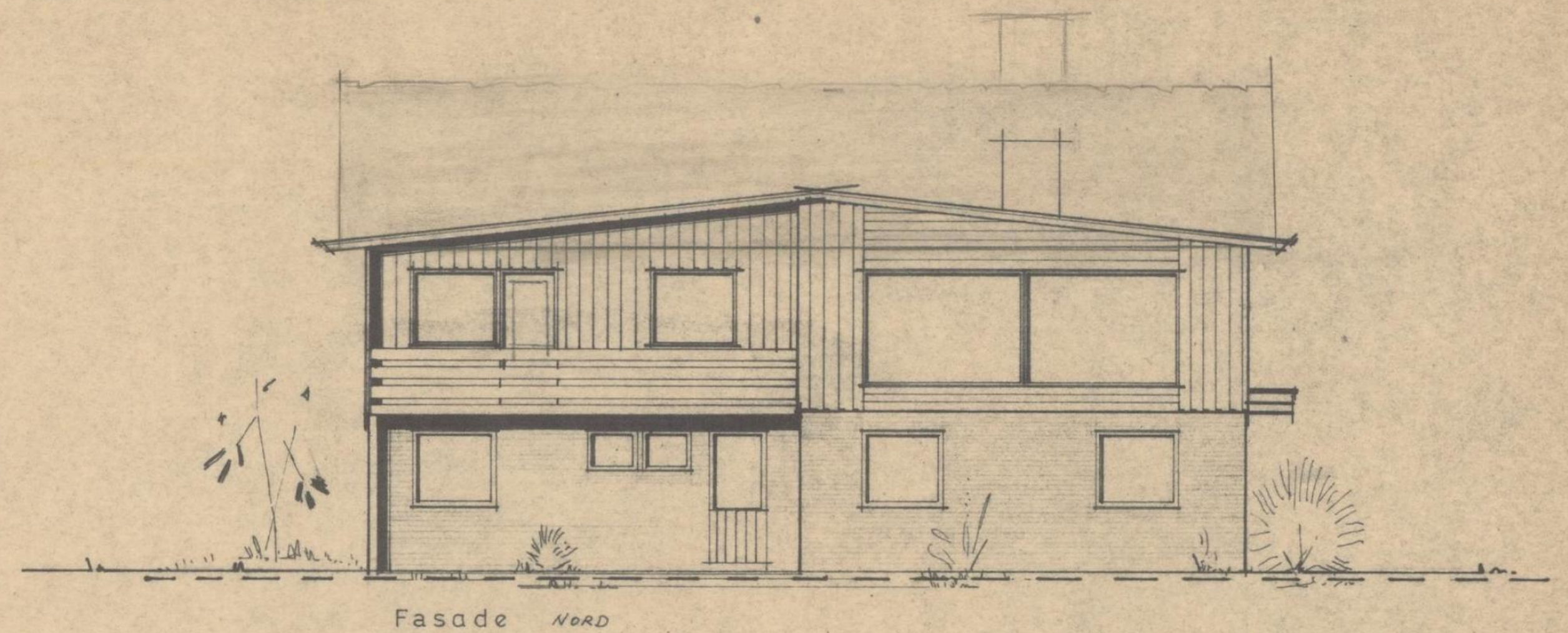
Fasade Nord
